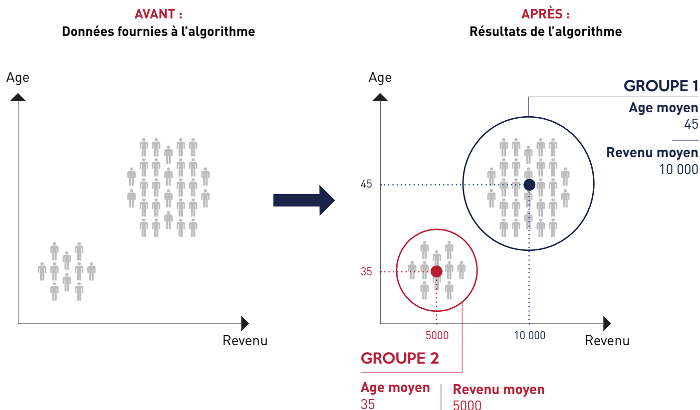
Figure : exemple fictif du fonctionnement de l'algorithme
